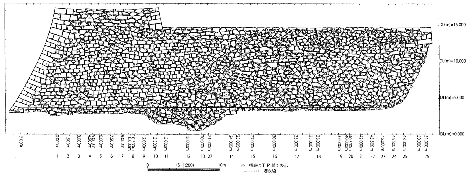
図4 北面石垣立面図
