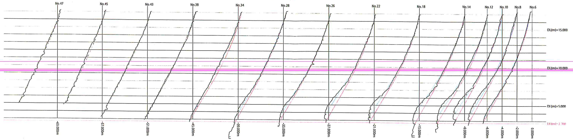
本丸搦手馬出東面断面図
