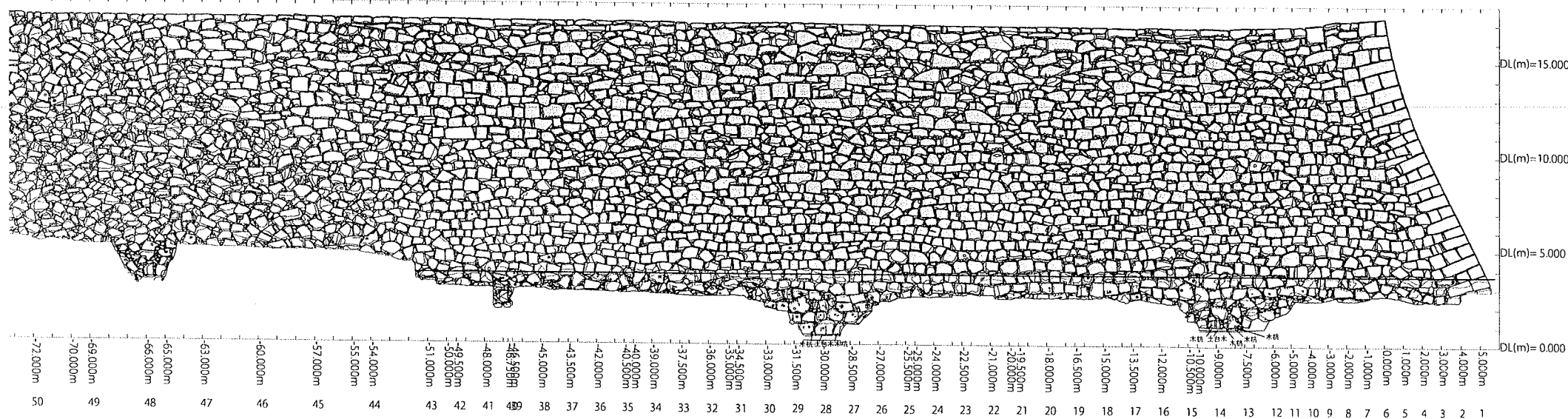
図3 東面石垣立面図
