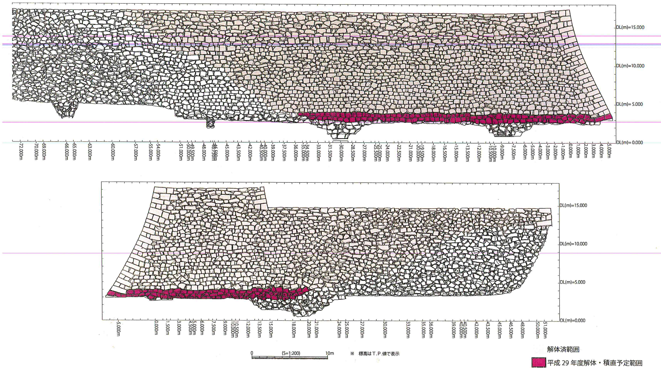
図 2 平成 29 年度石垣解体・積直予定範囲
